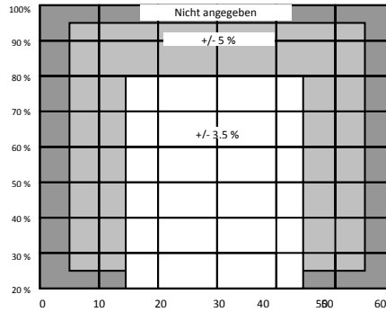
Grafik B: Genauigkeit der relativen Luftfeuchtigkeit
